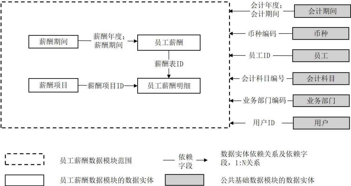
图1 员工薪酬数据实体关系
